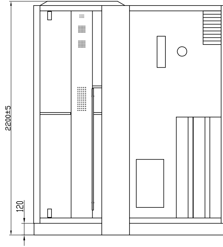
SR-89103RS 1800*1300*2200 (mm)
