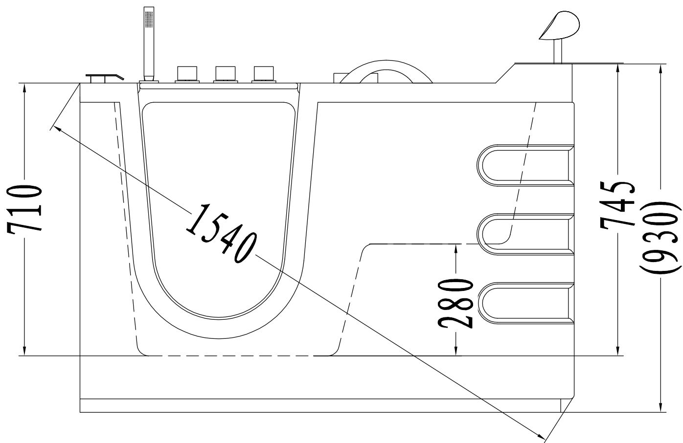
OLS-C106L线框图
